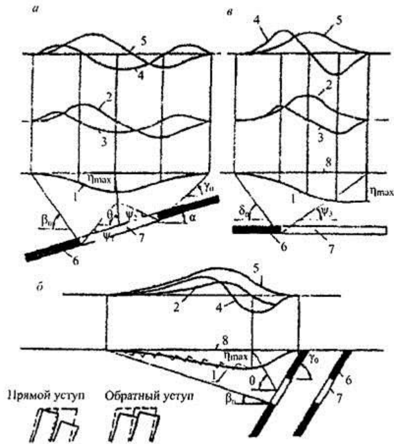
a - вертикальный разрез вкрест простирания при наклонном залегании угольных пластов; б - то же, при кругом залегании угольных пластов; в - вертикальный разрез по простиранию пластов; 1 - кривые оседаний; 2 - эпюры наклонов; 3 - эпюры кривизны; 4 - эпюры относительных горизонтальных деформаций; 5 - эпюры горизонтальных сдвижений; 6 - пласт; 7 - очистная выработка; 8 - положение земной поверхности до подработки; \eta_{\max} - максимальное оседание земной поверхности; \beta_0 , \gamma_0 , \delta_0 - граничные углы сдвижения; \psi_1 , \psi_2 , \psi_3 - углы полных сдвижений; \theta - угол максимального оседания; \alpha - угол падения пласта
