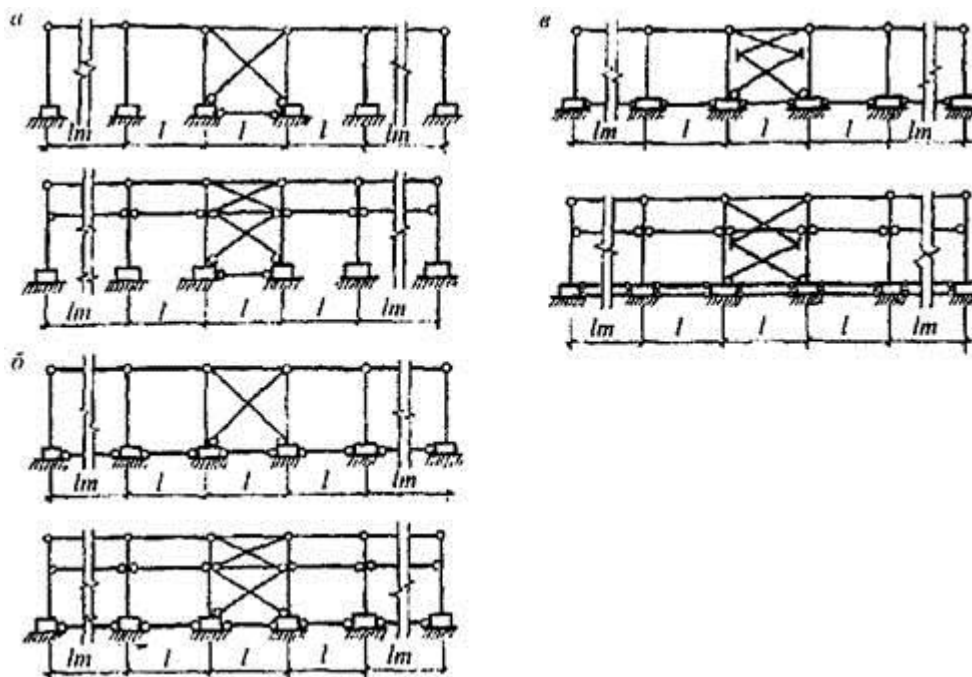
a - e - типы соединений элементов каркаса
