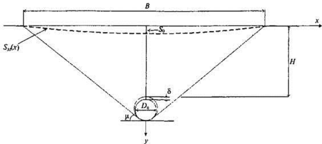
S_0 - значение максимального оседания поверхности основания под влиянием подземной выработки (как правило, над центром подземной полости); B - ширина мульды, т.е. расстояние между точками поверхности, в которых «оседание» поверхности равно нулю или минимальному значению, установленному в соответствии с проектными требованиями; H - глубина залегания,
