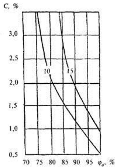
Рисунок Ш.5 - Изолинии сорбционного влагосодержания керамзитобетона \rho_0 = 1200 кг/м 3 , содержащего NaCl - 50 %, KCl - 30 %, MgCl 2 - 10 %, при изменении относительной влажности воздуха \phi_a , %, и массового солесодержания C , %, в стенах цехов дробления руды
