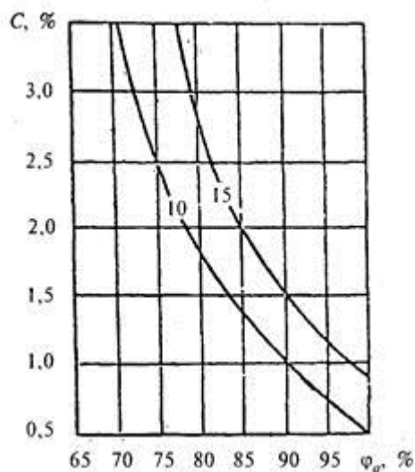
Рисунок Щ.1 - Изолинии сорбционного влагосодержания керамзитобетона \rho_0 = 1200 кг/м 3 , содержащего хлорид натрия, при изменении относительной влажности воздуха \varphi_a , %, и массового солесодержания C , %
