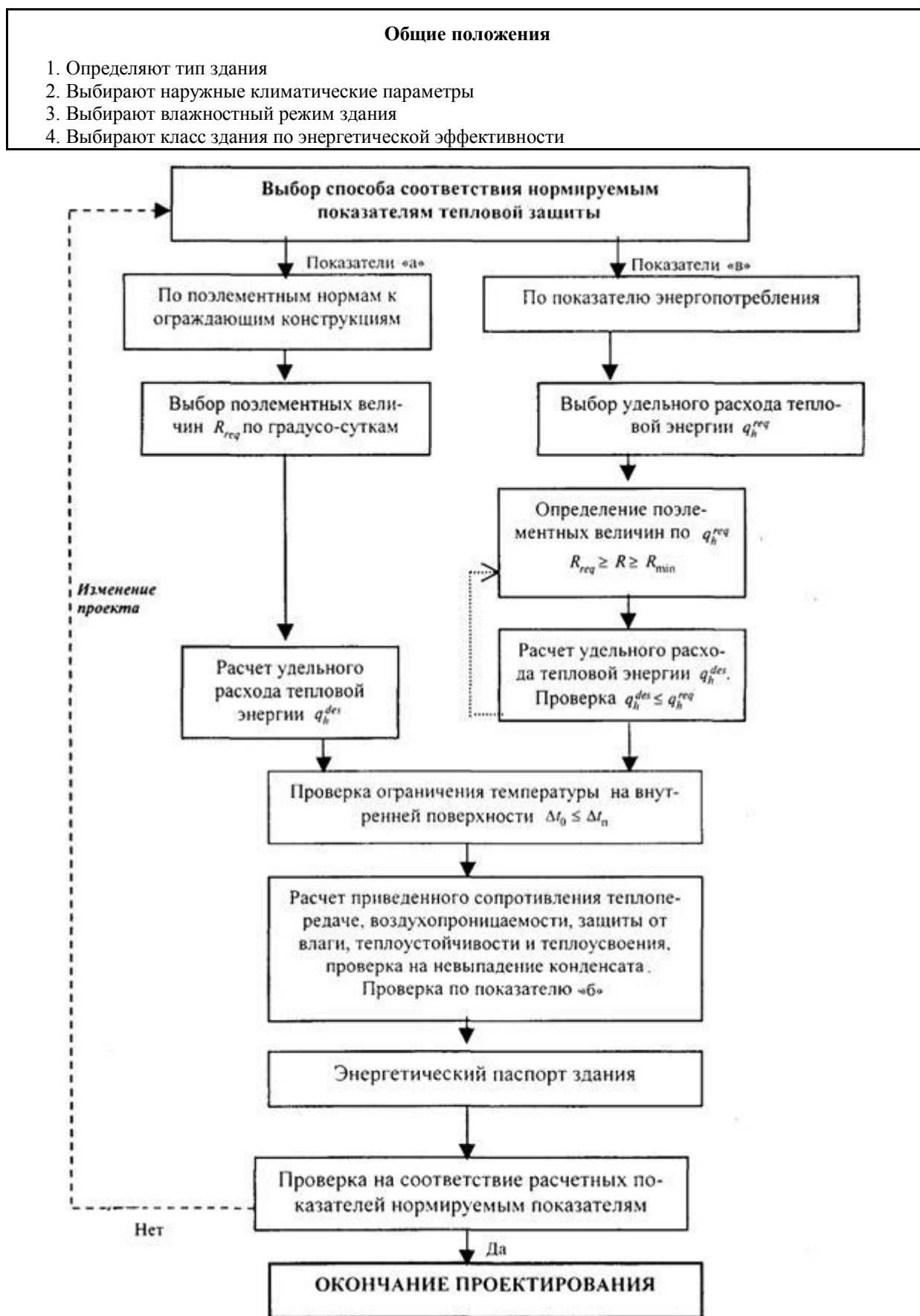
Рисунок 1 - Схема проектирования тепловой защиты зданий
