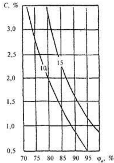
Рисунок Ш.4 - Изолинии сорбционного влагосодержания керамзитобетона \rho_0 = 1200 кг/м 3 , содержащего NaCl - 60 %, KCl - 30 %, MgCl 2 - 10 %, при изменении относительной влажности воздуха \phi_a , %, и массового солесодержания C , %, в стенах флотофабрик
