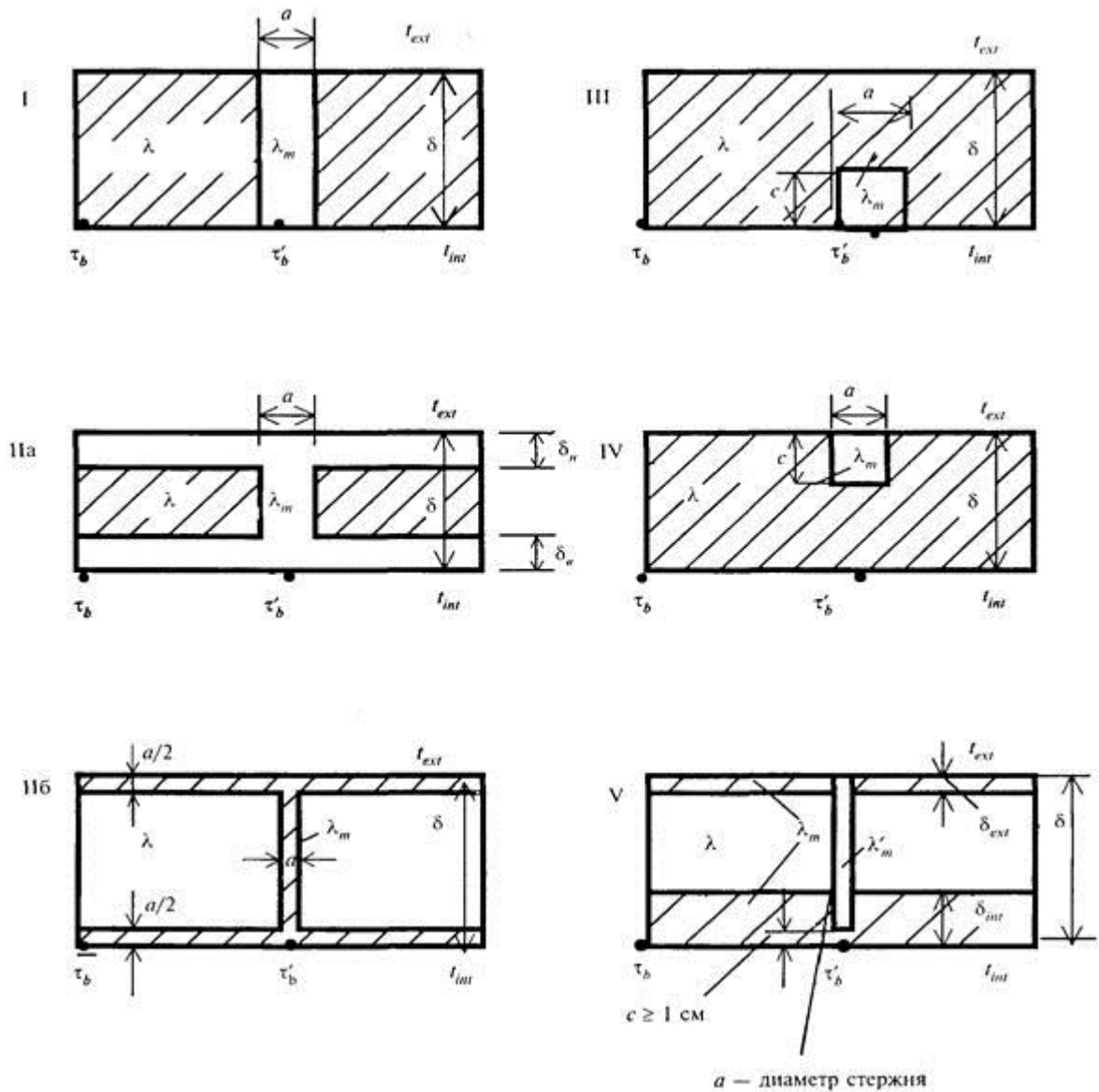
Рисунок Н.1 - Схемы теплопроводных включений в ограждающих конструкциях Н.1 РАСЧЕТ КОЭФФИЦИЕНТА ТЕПЛОТЕХНИЧЕСКОЙ ОДНОРОДНОСТИ k ПО ФОРМУЛЕ (12) НАСТОЯЩЕГО СВОДА ПРАВИЛ
