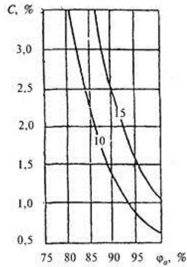
Рисунок III.2 - Изолинии сорбционного влагосодержания керамзитобетона \rho_0 = 1200 кг/м 3 , содержащего хлорид калия, при изменении относительной влажности воздуха \phi_a , %, и массового солесодержания C , %
