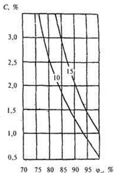
Рисунок III.6 - Изолинии сорбционного влагосодержания керамзитобетона \rho_0 = 1200 кг/м 3 , содержащего NaCl - 30 %, KCl - 60 %, MgCl 2 - 10 %, при изменении относительной влажности воздуха \phi_a , %, и массового солесодержания C , %, в стенах цехов сушки
