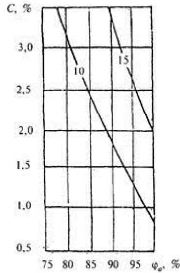
Рисунок III.3 - Изолинии сорбционного влагосодержания керамзитобетона \rho_0 = 1200 кг/м 3 , содержащего хлорид магния, при изменении относительной влажности воздуха \phi_a , %, и массового солесодержания C , %
